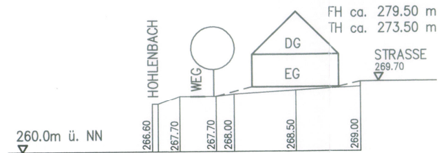
SCHNITT D-D
