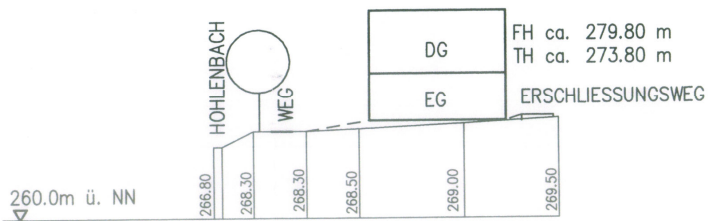
SCHNITT C-C
