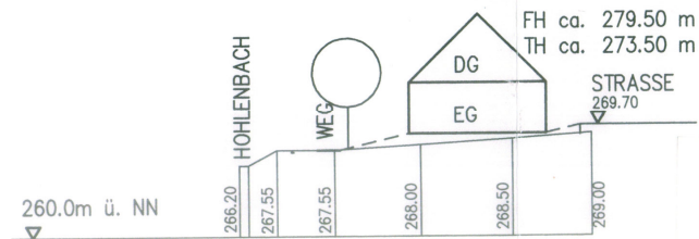
SCHNITT E-E
